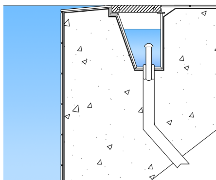
Bild 19. Finland skvalpräna (hög vattennivå med vågdämpning) Användningen av detta kantutföran- de innebär att vattenytan kommer att ligga i nivå med omkringliggande golvtytor.
