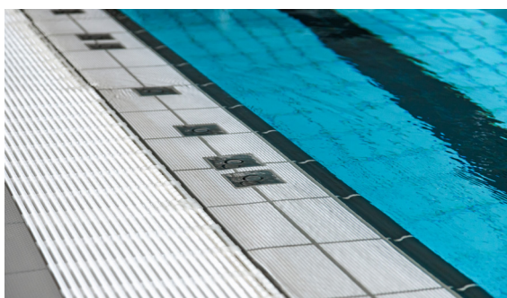
Bild 4. Rännor som kan beträddas måste täckas med galler som är avsedda för ändamålet. Öppningar i gallret får vara max 8 mm breda. Avstånd mellan gallerkant och kant på skvalpräanna får vara max 8 mm totalt.
