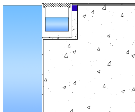
Bild 20. Wiesbaden skvalpräna (hög vattennivå utan vågdämpning) Denna kantlösning används då bas- sängens vattenyta önskas ligga i nivå eller strax ovanför omgivande golvtytor. Här ställs inga krav på den vågdäm- pande effekten, som en lutande kant ger.
